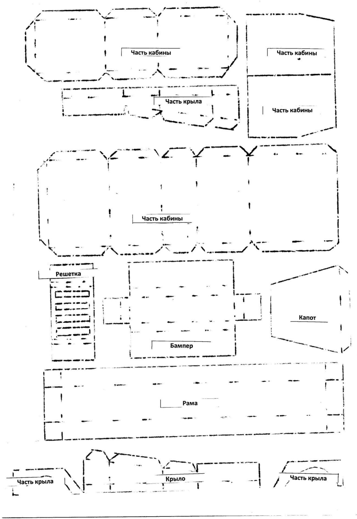
Чертеж автоцистерны
